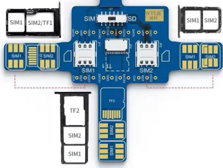
Placa de Teste Sinal de Smartphone Universal WYLIE
